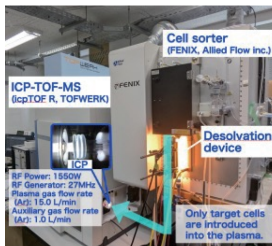
図 開発中の単一細胞内元素分析システム
