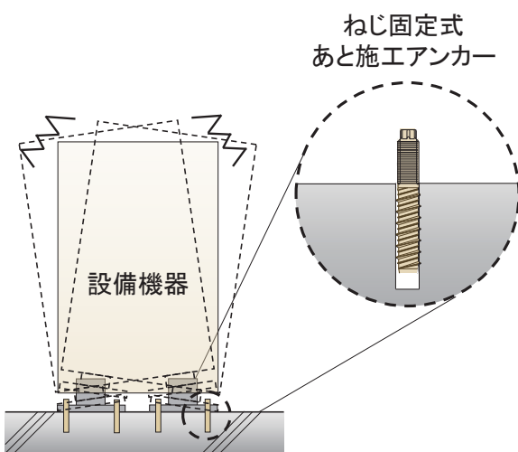
図1 あと施工アンカーの概要
