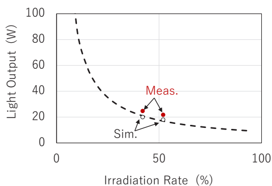
光源出力の連続走行条件
